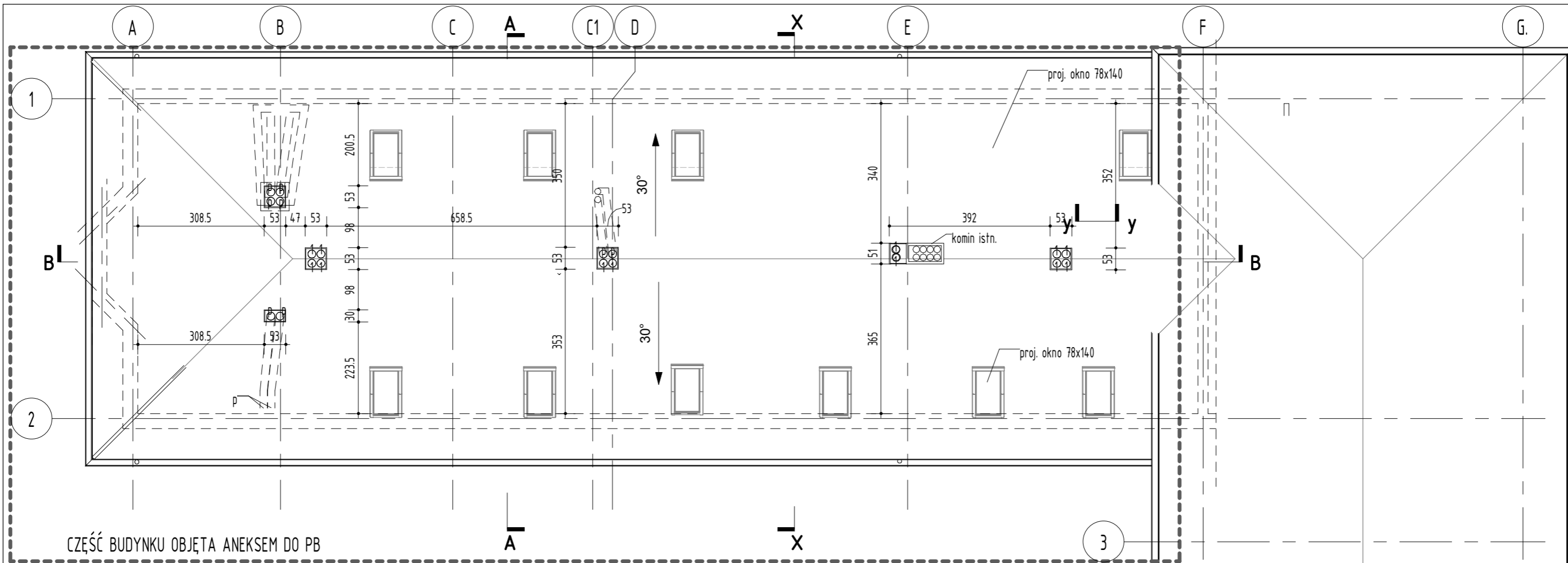
1 Rzut dachu 1 : 100
